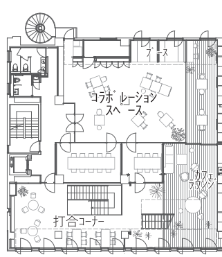
2 階平面図
